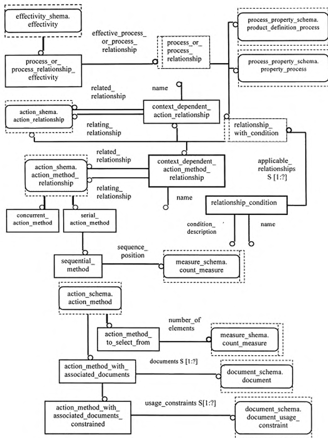
Рисунок D.1 — method_definition_schema — EXPRESS-G диаграмма 1 из 1
