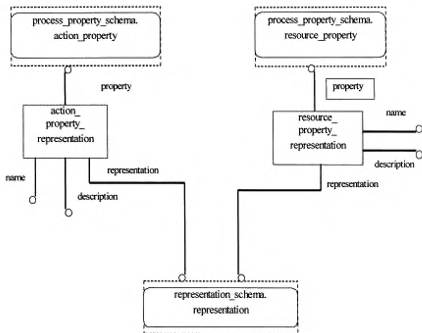
Рисунок D.3 — process_property_representation_schema — EXPRESS-G диаграмма 1 из 1
