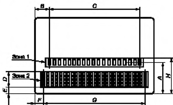
Рисунок 1 — Расположение зон тиснения
