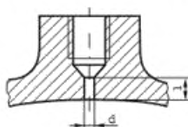
Рисунок 8 – Пример разъема для измерения давления
