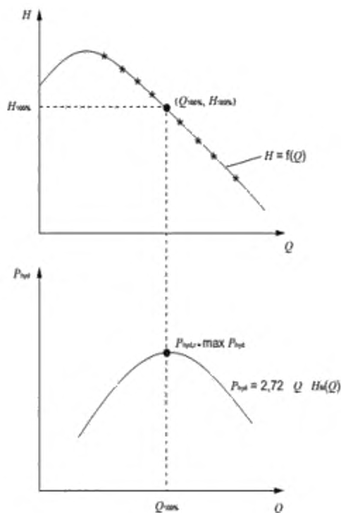
Рисунок 2 – Номинальная гидравлическая мощность на выходе
