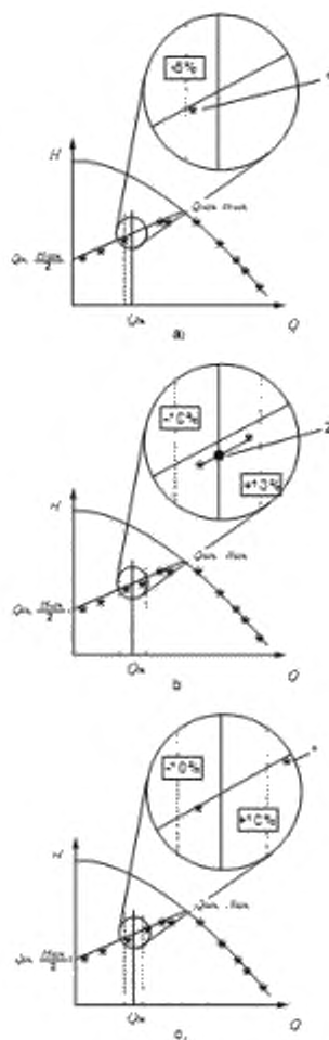
Рисунок 5 – Правила интерполяции
