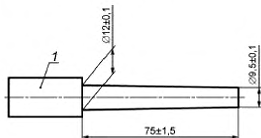
Рисунок Г.1 — Размеры испытательного штифта
