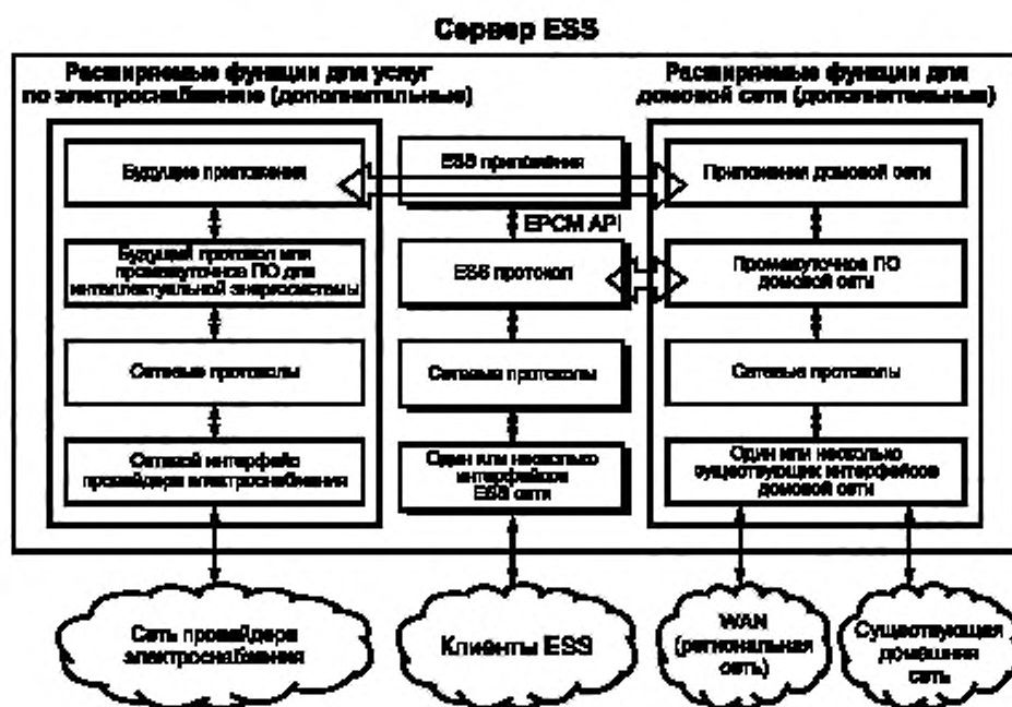
Рисунок 2 — Основные ESS и его возможное расширение
