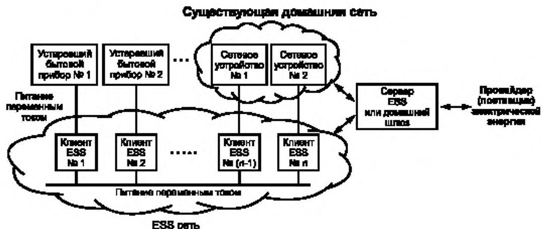
Рисунок 1 — Архитектура системы энергосбережения
