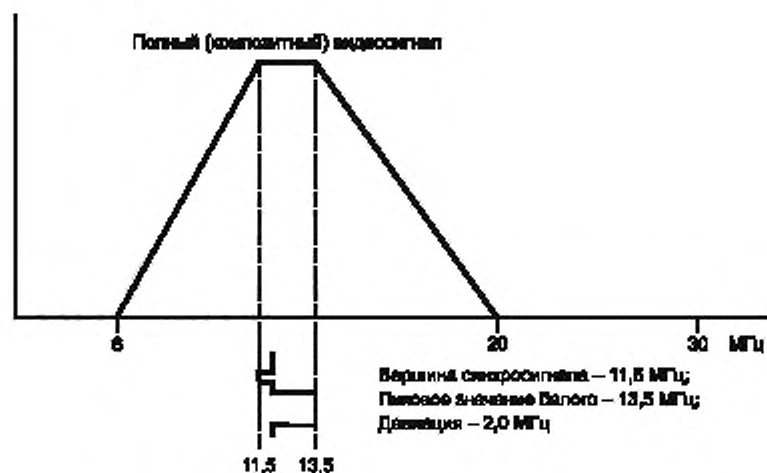
Рисунок 12 — Формат передачи [полный (композитный) видеосигнал]
