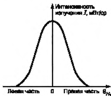
8a — Направленность по горизонтали
