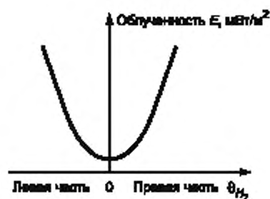
10a — Направленность по горизонтали
