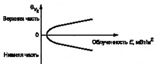
10b — Направленность по вертикали
