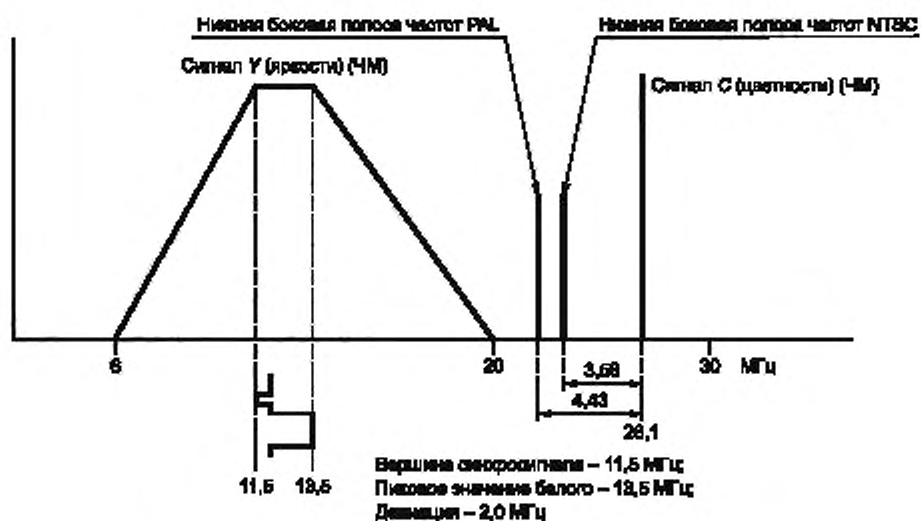
Рисунок 13 — Формат передачи (видеосигнал Y/C с разделением)
