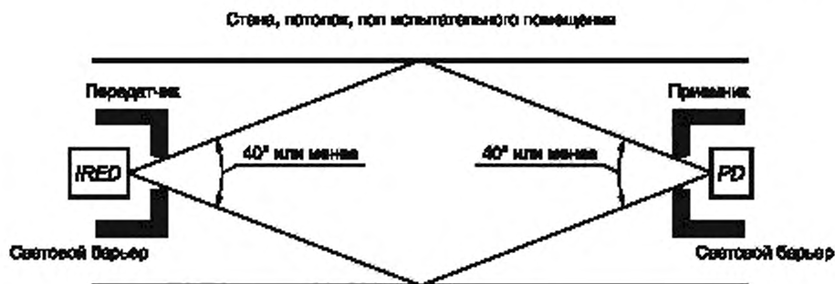
Рисунок 2 — Размещение при измерении
