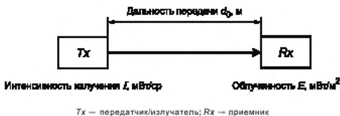
Рисунок 3 — Дальность передачи
