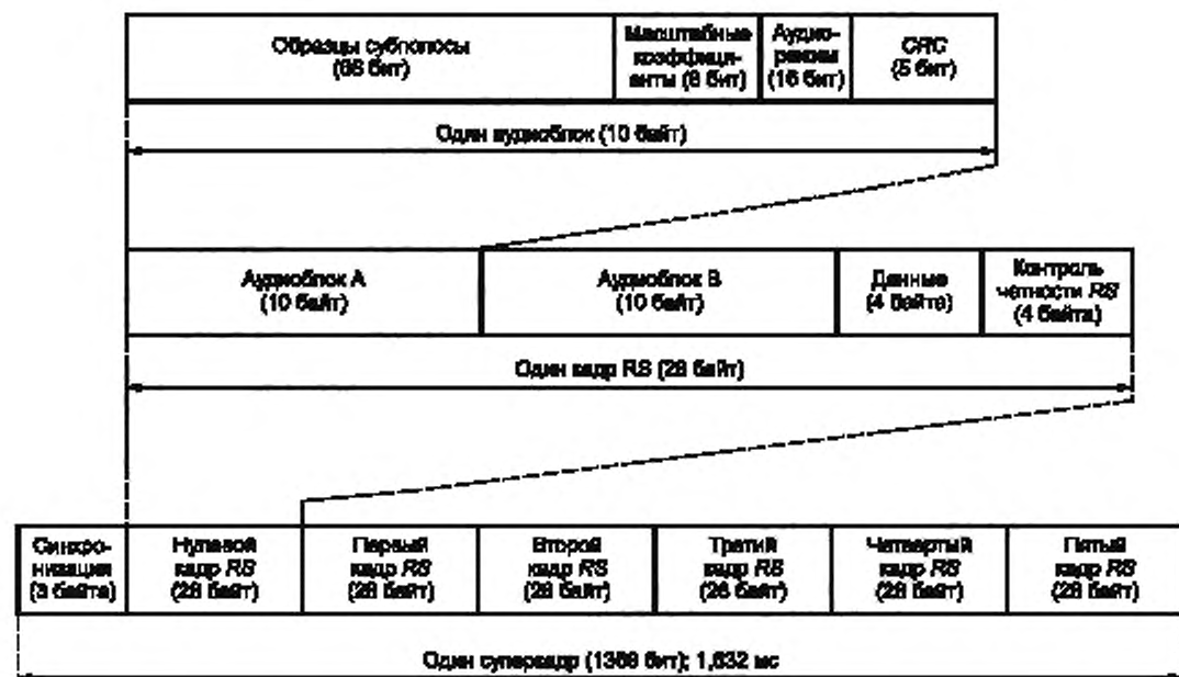
Рисунок 9 — Структура суперкадра
