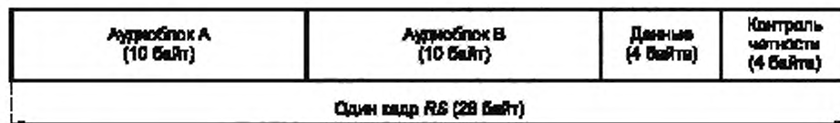
Рисунок 10 — Структура RS -кадра
