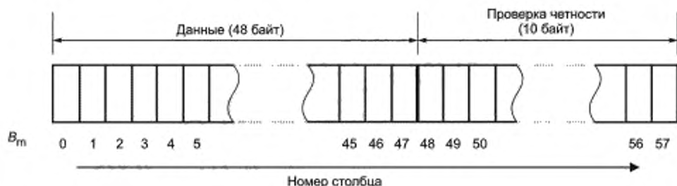
Рисунок 13 — Блок кода коррекции ошибки
