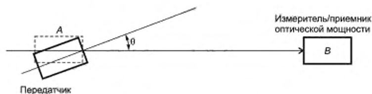
Рисунок 28 — Характеристики передатчика
