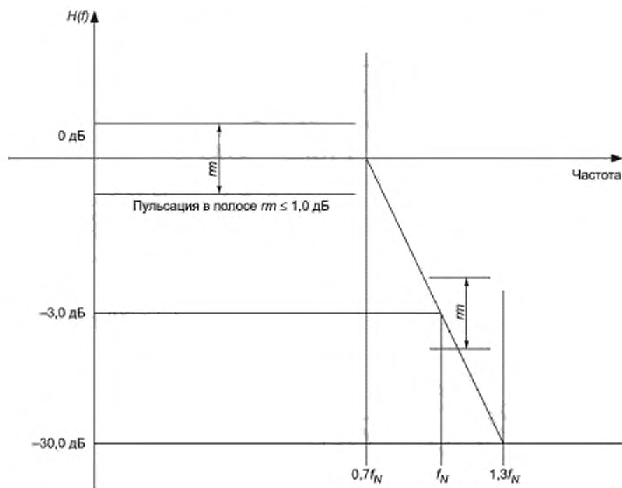
Рисунок 21 — Характеристики фильтра основной полосы
