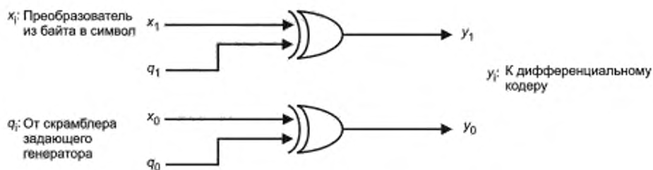
Рисунок 18 — Логические элементы «исключающие ИЛИ» ( XOR )
