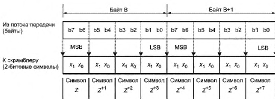
Рисунок 17 — Преобразование байта в символ
