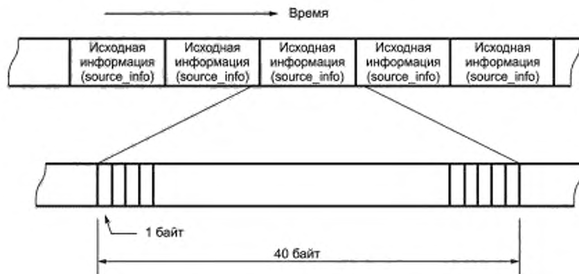
Рисунок 10 — Поток исходной информации (source_info stream)
