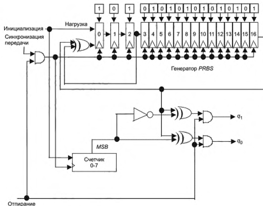
Рисунок 19 — Задающий генератор скремблера
