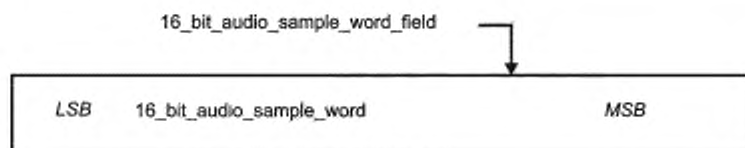
Рисунок В.5 — Структура субкадра режима половины полосы
