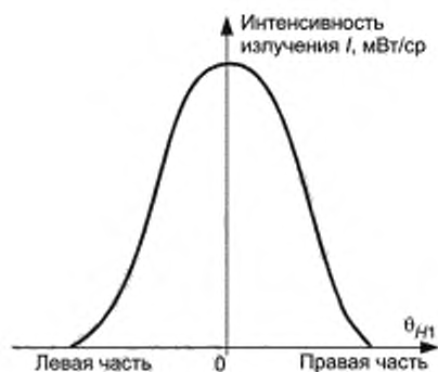
Рисунок 29а — Направленность по горизонтали
