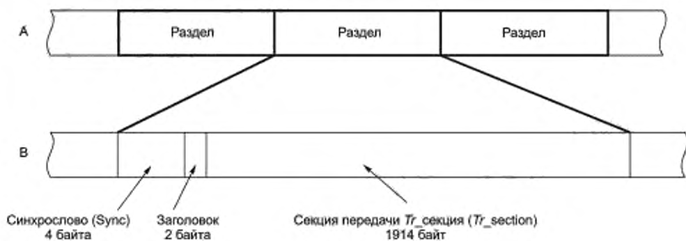
Рисунок 14 — Поток передачи
