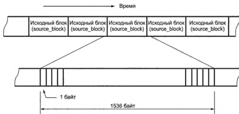
Рисунок 9 — Поток исходных блоков (source_block stream)
