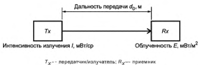
Рисунок 24 — Дальность передачи
