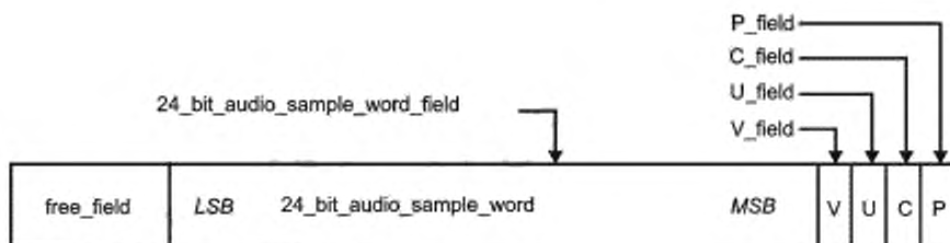
Рисунок В.4 — Структура субкадра режима полной полосы
