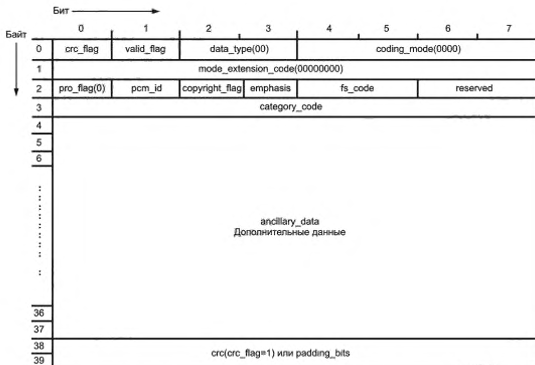
Рисунок А.1 — Структура исходной информации (source_info)
