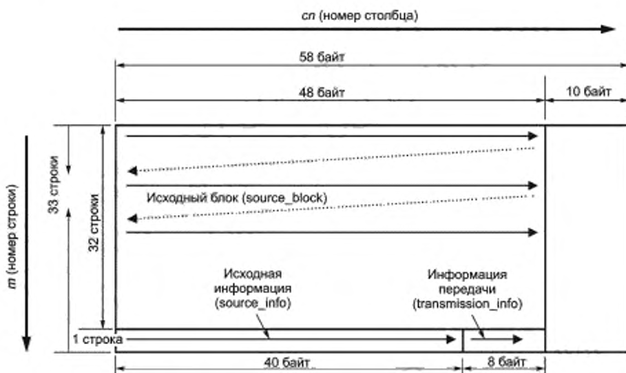
Рисунок 11 — Размещение в структуре блока (block_structure)
