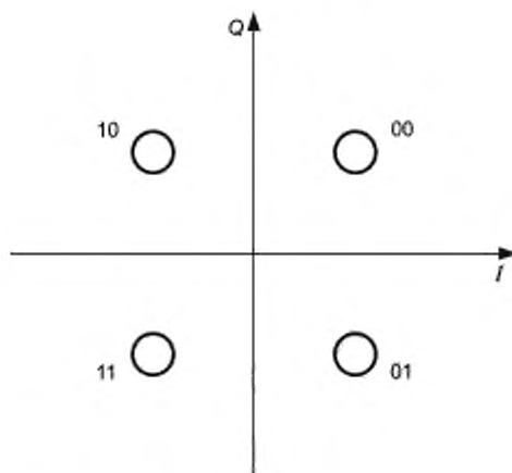
Рисунок 20 — Представление/топография QPSK
