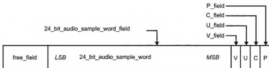
Рисунок А.4 — Структура субкадра режима полной полосы
