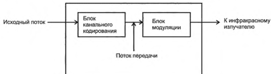
Рисунок 4 — Передатчик
