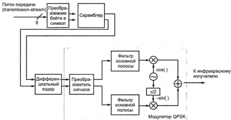
Рисунок 16 — Блок модуляции
