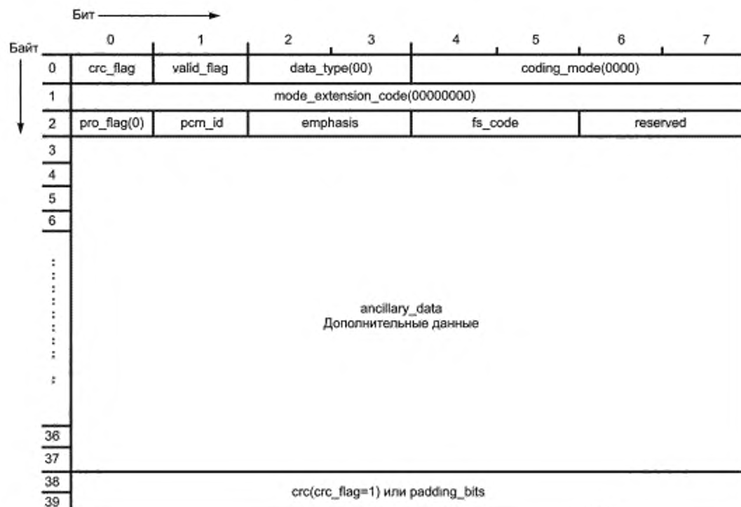
Рисунок В.1 — Структура исходной информации
