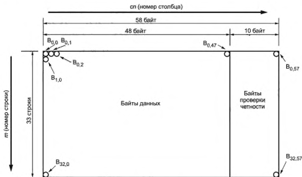
Рисунок 7 — Структура блока
