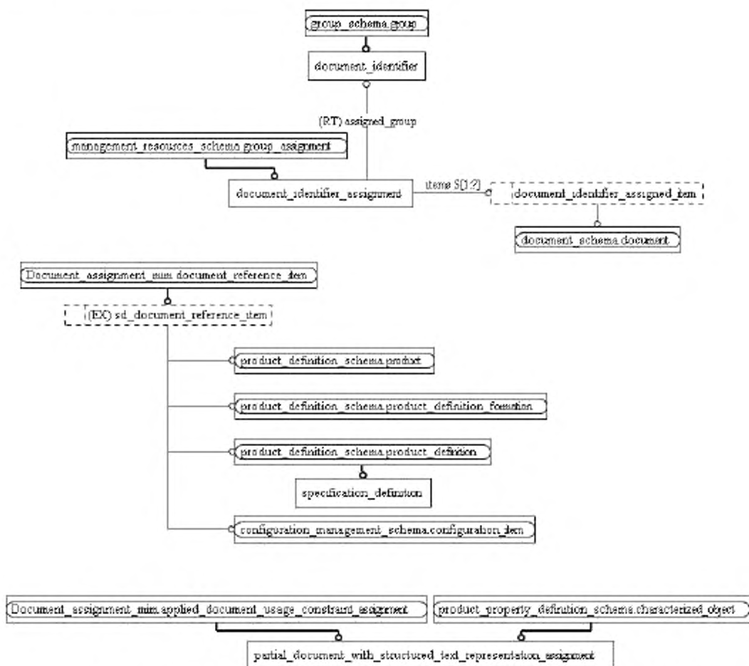
Рисунок D.2 – Представление IMM на уровне объектов в формате EXPRESS-G (диаграмма 1 из 1)
