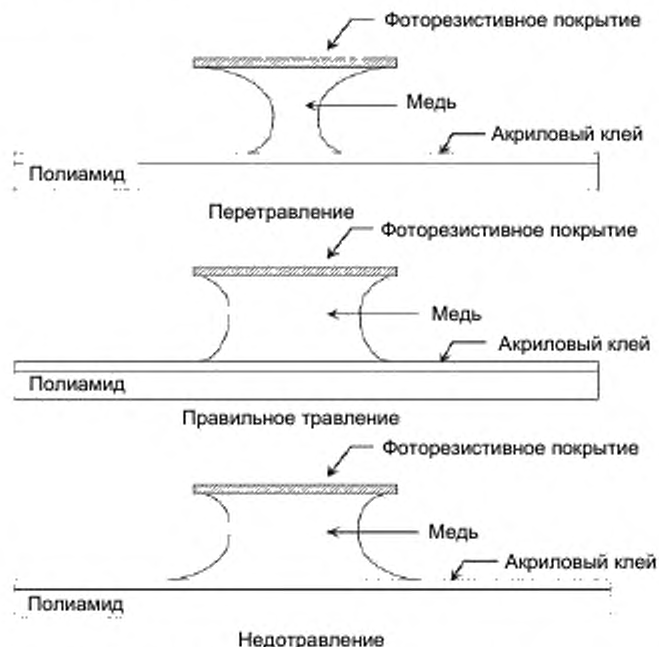
Рисунок 1 – Описание технологического процесса травления
