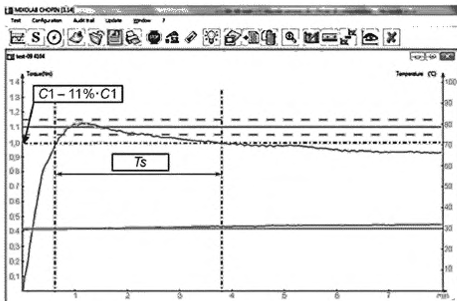
Рисунок А.2 — Расположение значений времени T_1 и температуры теста на кривой «Микосаба»
