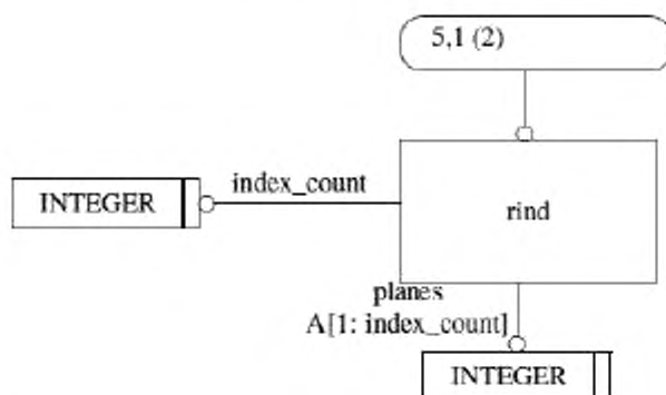
Рисунок D.5 — Представление схемы mesh_toplogy_schema на уровне объектов в формате EXPRESS-G (5 из 10)
