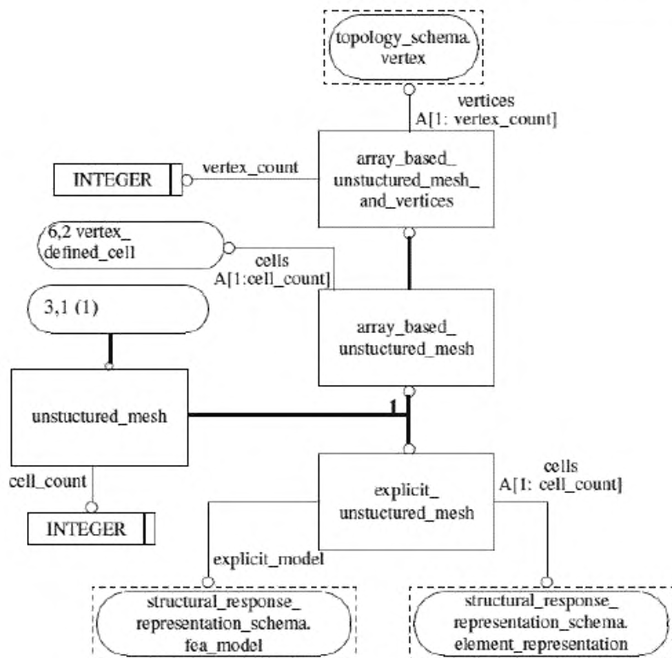
Рисунок D.3 — Представление схемы mesh_topology_schema на уровне объектов в формате EXPRESS-G (3 из 10)
