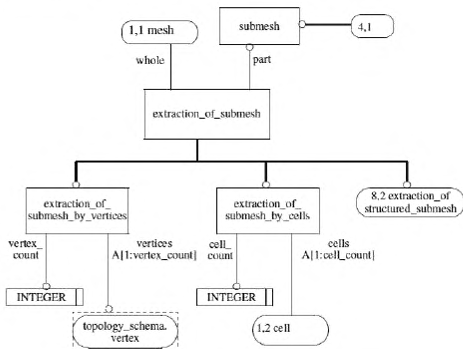
Рисунок D.4 — Представление схемы mesh_toplogy_schema на уровне объектов в формате EXPRESS-G (4 из 10)
