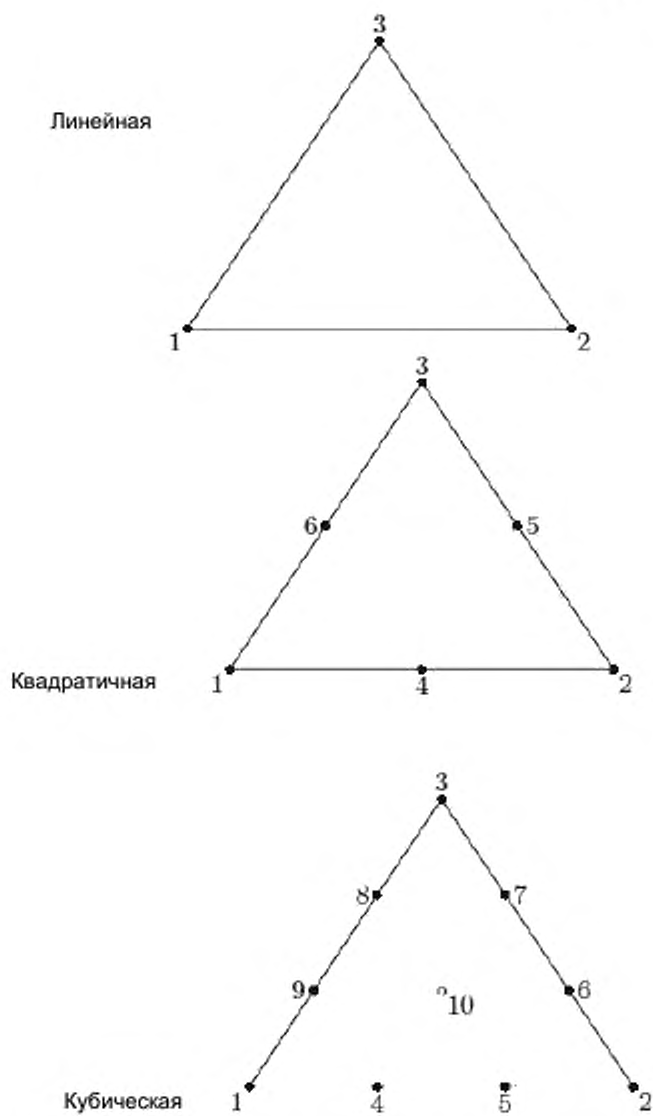
Рисунок 15 — Линейные, квадратичные и кубические треугольные ячейки
