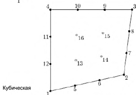
Рисунок 16 — Линейные, квадратичные и кубические четырехугольные ячейки
