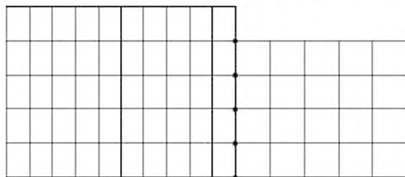
Рисунок 21 — Граничащий стык один к одному
