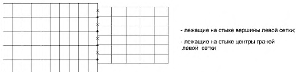
Рисунок 22 — Рассогласованный граничный стык
