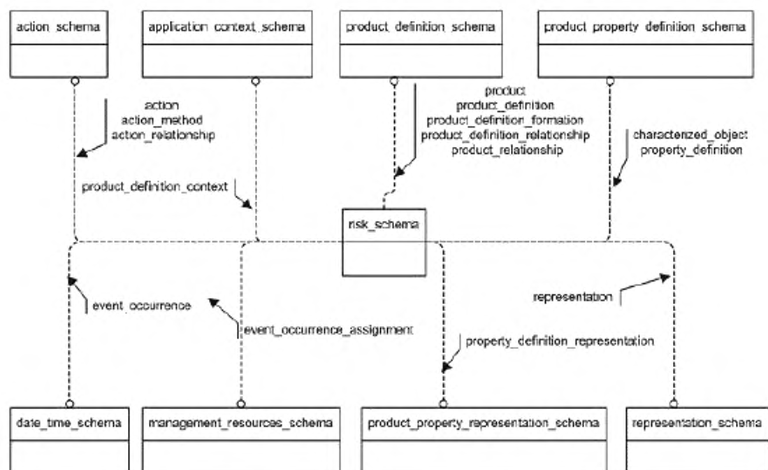
Рисунок 1 — Взаимосвязи между схемами в настоящем стандарте
