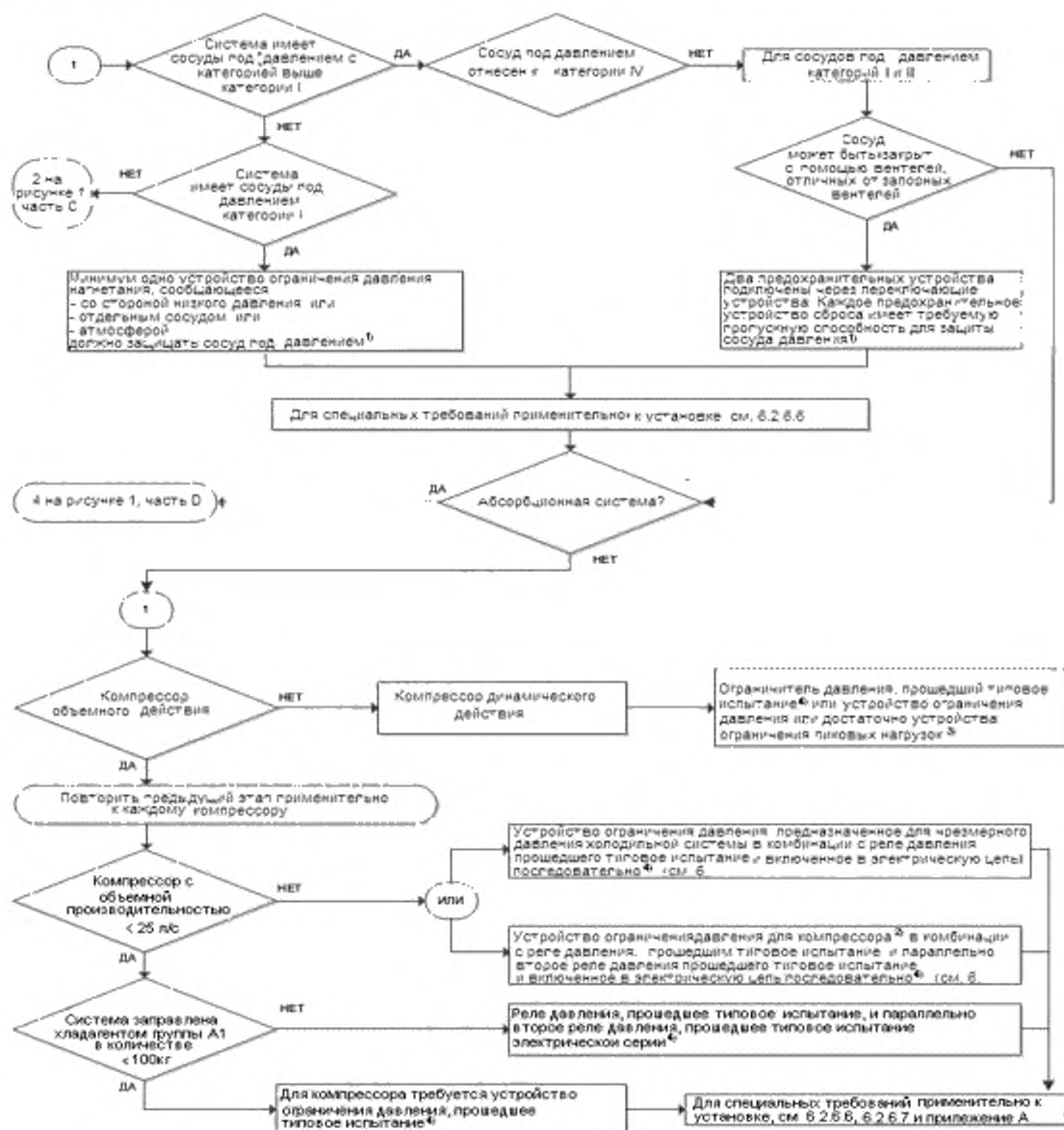
Рисунок 1, часть B – Защита холодильной системы от чрезмерного давления
