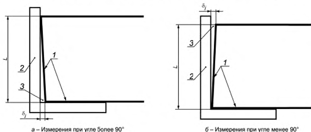
1 — сопрягаемые грани бортового камня; 2 — поверочный угольник 90°; 3 — максимальный зазор \delta_j , измеряемый на расстоянии L
