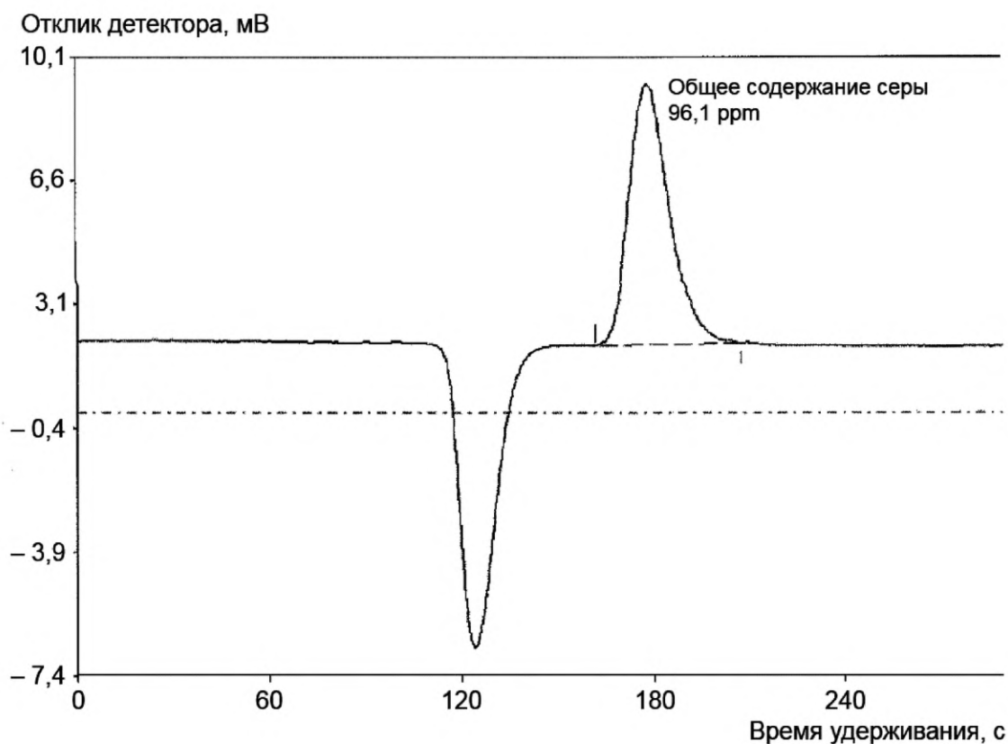
Рисунок 1 — Типовая хроматограмма
