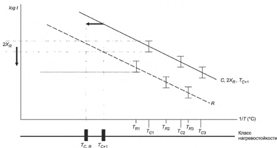
Рисунок 4 — Испытуемая система, аттестованная для другого срока эксплуатации и другого класса нагревостойкости по сравнению с эталонной
