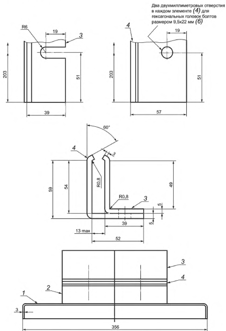
Рисунок А.2 — Типичный монтаж паза
