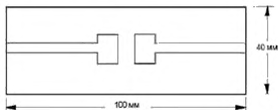
Рисунок F.1 — Пример испытываемой подложки в испытании, представленном таблицей F.1
