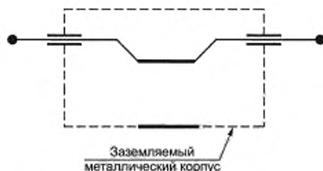
Рисунок 4b — Проходной конденсатор для асимметричного использования (некоаксиальный)
