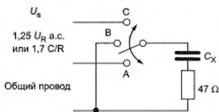
Рисунок В.1 — Цепь для испытания на долговечность
