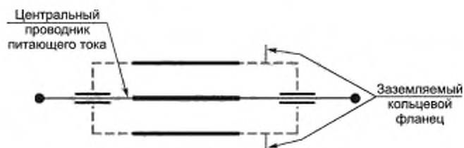
Рисунок 3 — Коаксиальный проходной конденсатор
