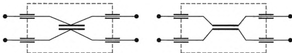
Рисунок 4а — Проходной конденсатор для симметричного использования (некоаксиальный)
