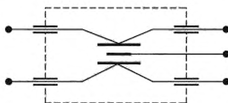
Рисунок 4d — Многозвенный проходной конденсатор
