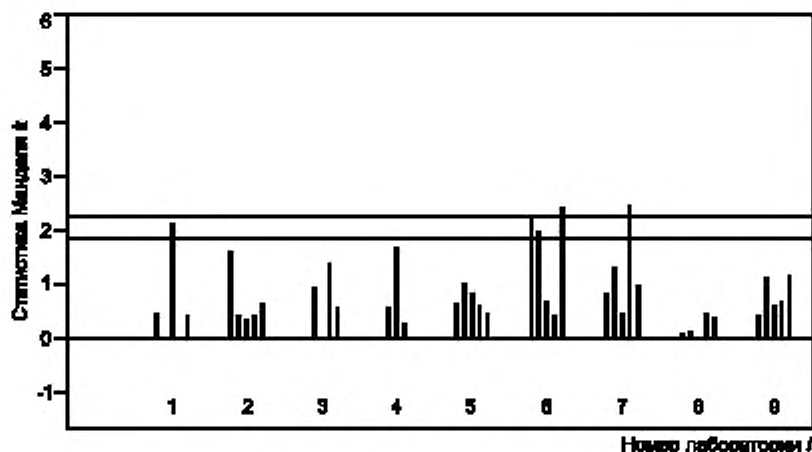
Рисунок В.8 — Титрование креозотового масла. Значения статистики внутрилабораторной совместимости Мандела k , сгруппированные по лабораториям
