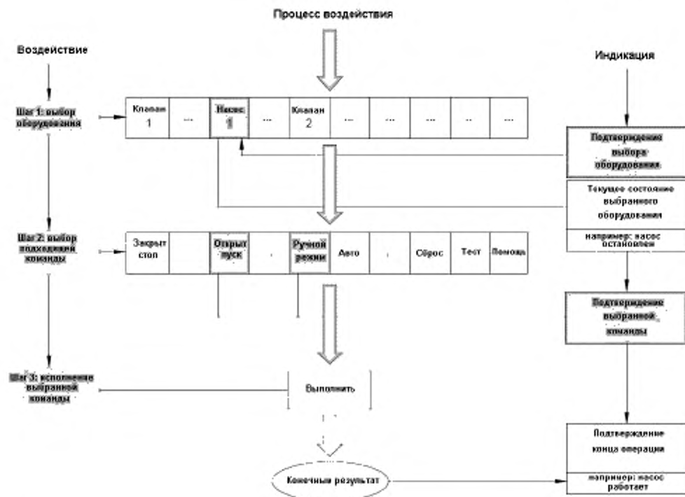
Рисунок 2 — Трехшаговая последовательность пуска для многофункционального применения
