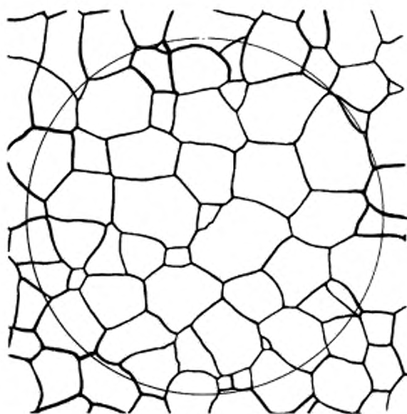
Рисунок В.2 — Зерна без двойников (равномерное травление)
