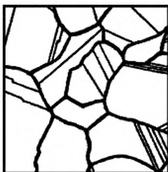
— Границы зерен
