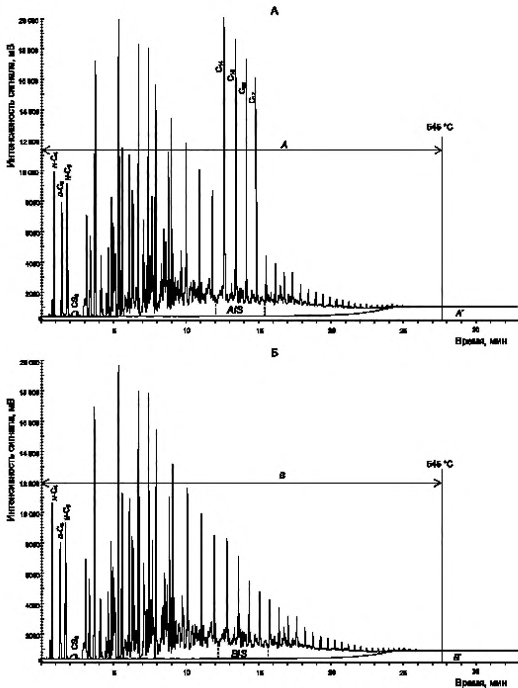
Рисунок 4 — Типовые хроматограммы стабильного газового конденсата (СГК)
