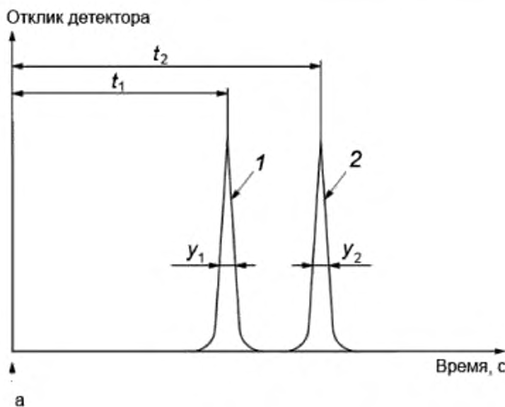
1 — гексадекан; 2 — октадекан; а — ввод пробы
