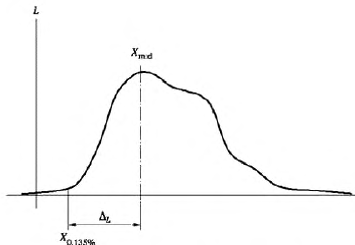
Рисунок 11 — Графическое представление метода вычисления \Delta_L
