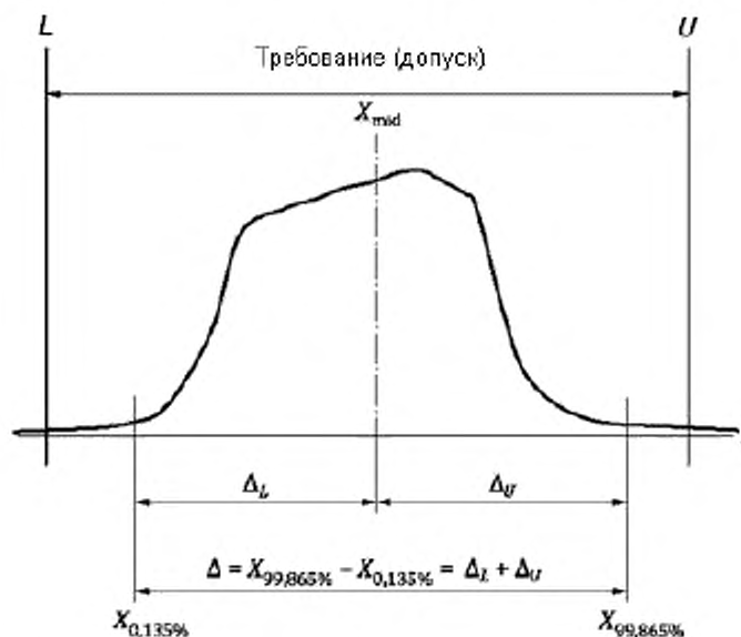
Рисунок 9 — Графическое представление общего геометрического метода
