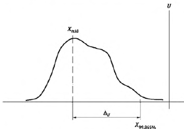
Рисунок 10 — Графическое представление метода вычисления \Delta_U
