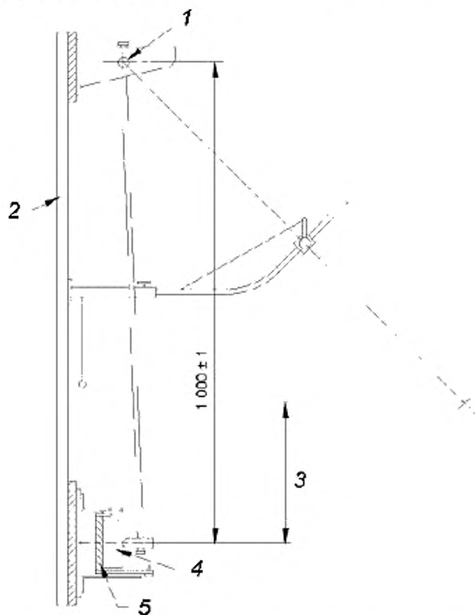
Рисунок 1 — Маятниковый стенд для испытаний на ударные воздействия
