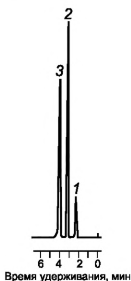
Рисунок 2 — Типовая хроматограмма сернистых соединений в нефти на колонке с 2 % ОДПН на диатомитовом кирпиче
