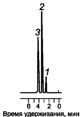
Рисунок 3 — Типовая хроматограмма сернистых соединений в нефти на колонке с 2 % ТБЦЭП на диатомитовом кирпиче
