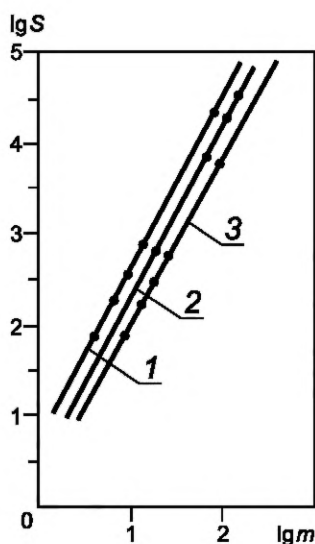
lg S — десятичный логарифм площади пика ССС; lg m — десятичный логарифм массы ССС; 1 — сероводород; 2 — метилмеркаптан; 3 — этилмеркаптан
