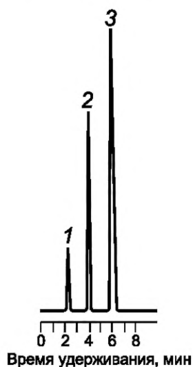
Рисунок 3 — Типовая хроматограмма сернистых соединений в нефти на колонке с 2 % ТБЦЭП на диатомитовом кирпиче
