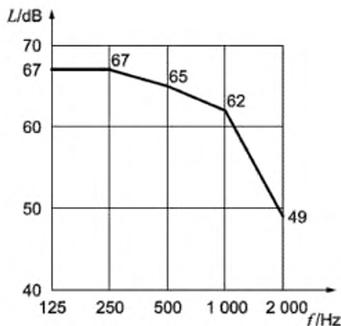
Рисунок 2 — Оценочная кривая для ударного шума (октавные полосы)
