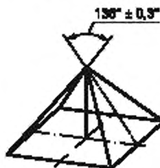
Рисунок 2 — Угол алмазной пирамиды Викерса
