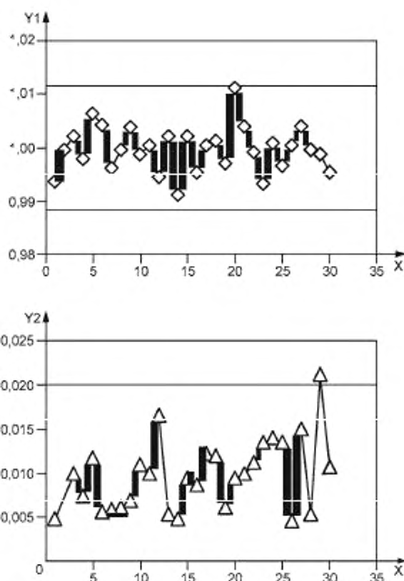
Y1 — среднее значение, мкм, при 0,1F_{max} ; Y2 — стандартное отклонение, мкм; X — количество косвенных проверок
