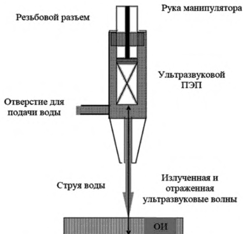
Рисунок 1 — Метод А. Автоматизированный ультразвуковой эхо-импульсный метод
