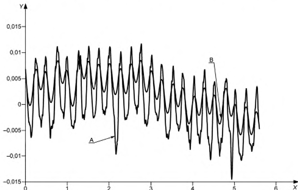
Рисунок A.6 — Исходный профиль
