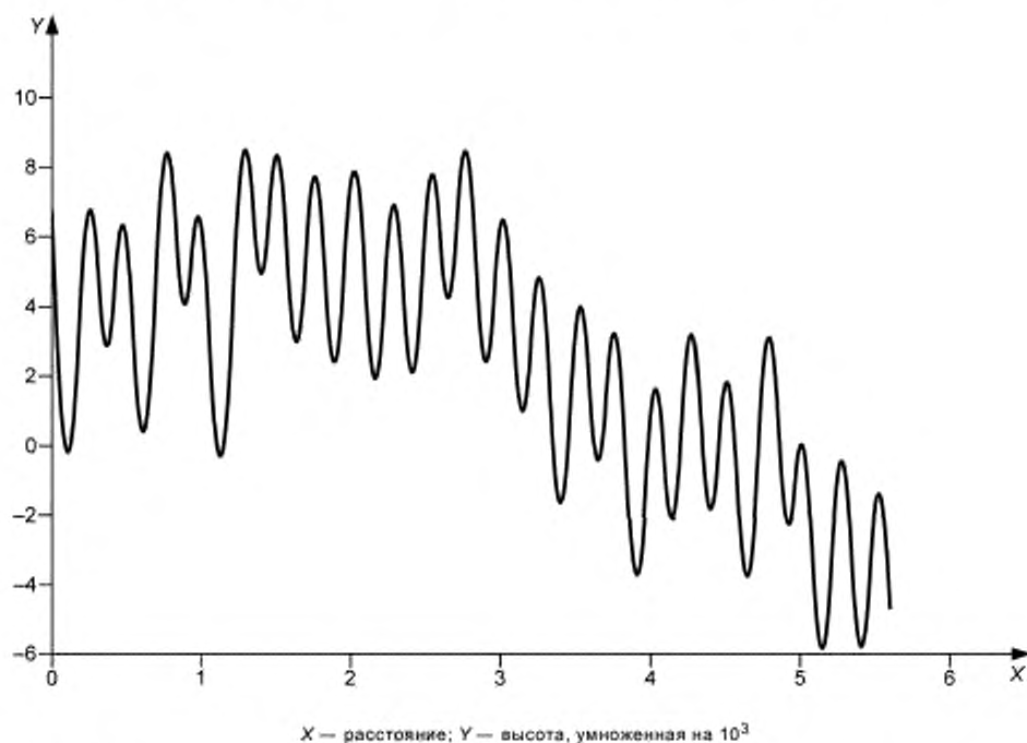
Рисунок А.5 — Пример первичной математической модели с радиусом вложенного индекса 0,8 мм
