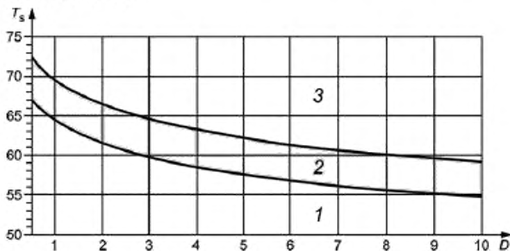
Рисунок 2 — Область разброса порога возникновения ожога при контакте кожи с горячей гладкой поверхностью металла без покрытия
