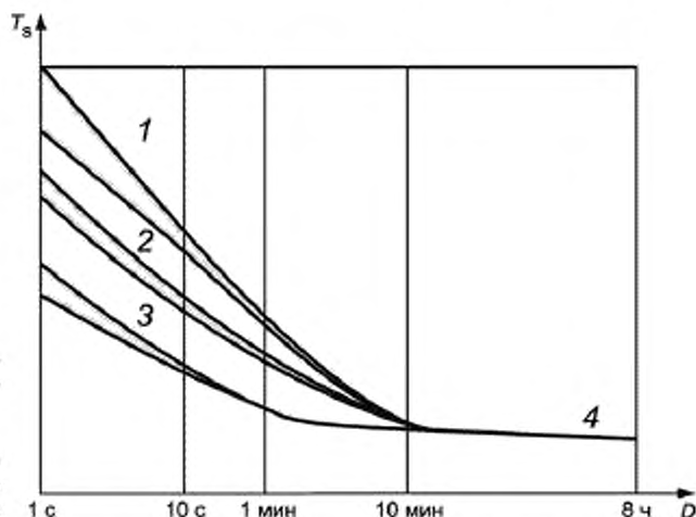
Рисунок 1 — Взаимосвязь между порогом возникновения ожога и периодом контакта при контакте кожи с горячей поверхностью
