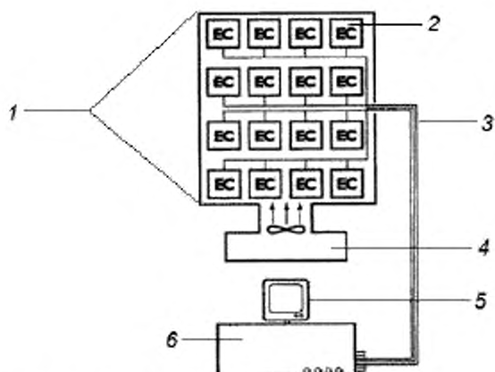
1 — плоскость испытания 1220 × 1830 мм; 2 — стекла с ЭХП; 3 — электрические выводы и кабели терморпар; 4 — термощаф; 5 — компьютер; 6 — многоканальная цифровая автоматизированная система управления и сбора данных
