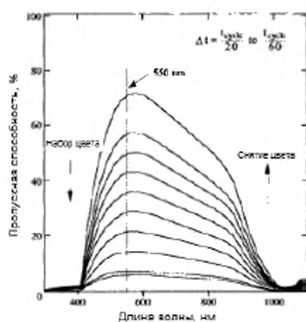
Рисунок 4 — Типовые спектры пропускания
