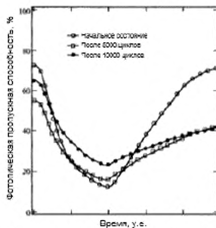
Рисунок 5 — Фотометрическая пропускная способность как функция времени, измеренного на различных этапах циклических испытаний типового окна с ЭХП
