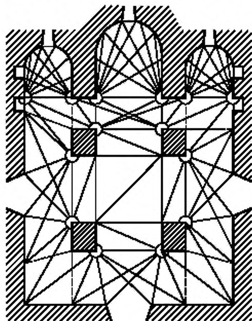
Рисунок Б.1 — Схема обмера плана методом триангуляции
