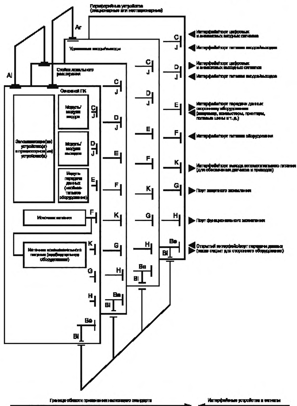
Рисунок 3 — Типовая конфигурация интерфейсов/портов ПЛК-системы, лист 1 (по МЭК 61131-2)
