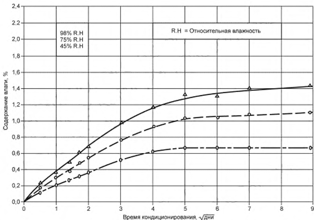
Рисунок 1 — Пример графика влагопоглощения углерод/эпоксидных (0,45—45,0) 5 слоистых материалов из восьми слоев при температуре 48,9 °С (8)
