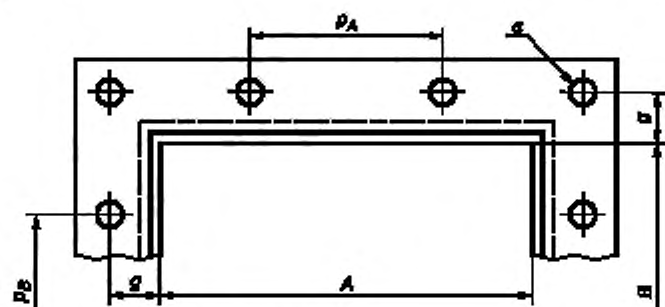
Приваренный внахлест фланец
