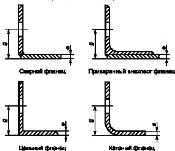
Рисунок 4 — Размеры и способы изготовления прямоугольных фланцев
