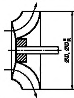
Рисунок 3 — Рабочее колесо диагонального вентилятора
