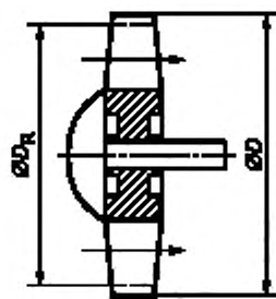
Рисунок 2 — Рабочее колесо осевого вентилятора
