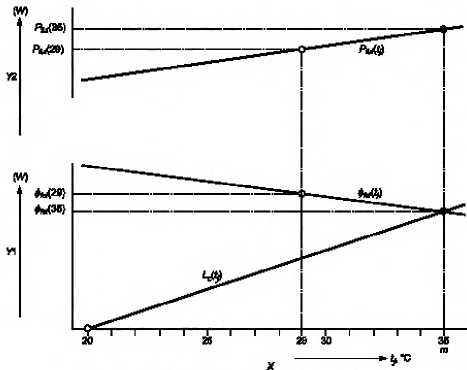
Рисунок А.1 — Холодопроизводительность, потребляемая мощность и нагрузка охлаждения для установок с нерегулируемой производительностью
