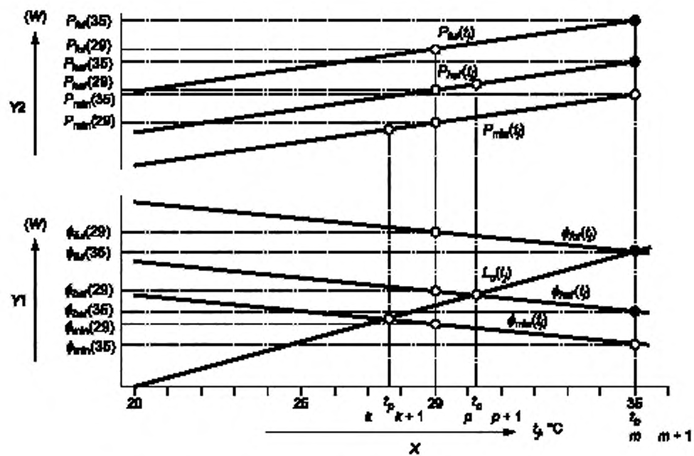
Рисунок А.3 — Холодопроизводительность, потребляемая мощность и нагрузка охлаждения для установок с многоступенчатой производительностью
