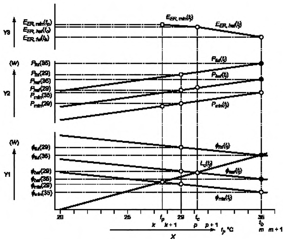
Рисунок А.4 — Холодопроизводительность, потребляемая мощность, нагрузка охлаждения и EER для установок с регулируемой производительностью
