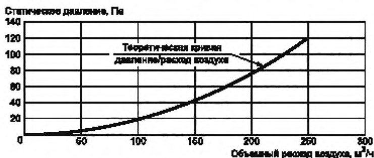
Рисунок В.1 — Кривая давление/объемный расход воздуха
