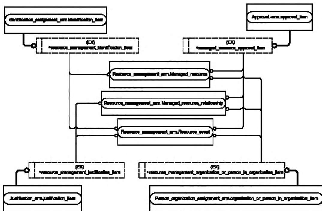
Рисунок С.3 — Представление ПЭМ на уровне объектов в формате EXPRESS-G (диаграмма 2 из 4)
