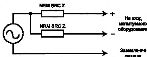
Рисунок 34 — Метод измерения коэффициента подавления синфазного сигнала
