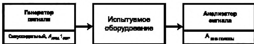
Рисунок 30 — Метод измерения подавления компонентов отображения
