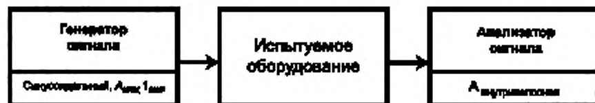
Рисунок 29 — Метод измерения подавления составляющих искажения
