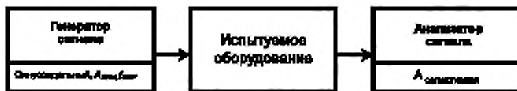
Рисунок 9 — Метод измерения амплитудно-частотных характеристик
