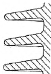
Рисунок 3б — Аэродинамические ребра — длинностержневые, опорные и полые изоляторы
