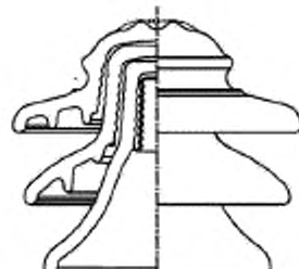
Рисунок 6б — Многоэлементный штыревой изолятор
