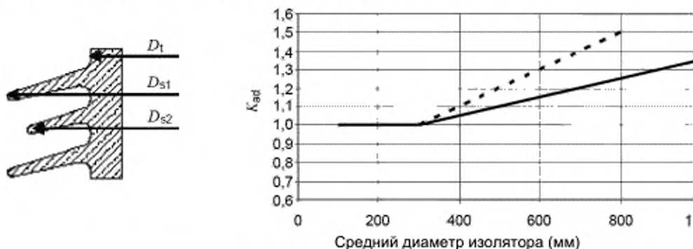
Рисунок 16 — K_{agr} в зависимости от диаметра изолятора
