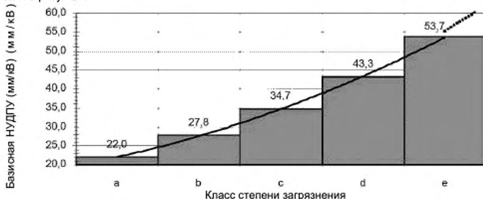
Рисунок 1 — БНУДПУ в функции от класса СЗЭ
