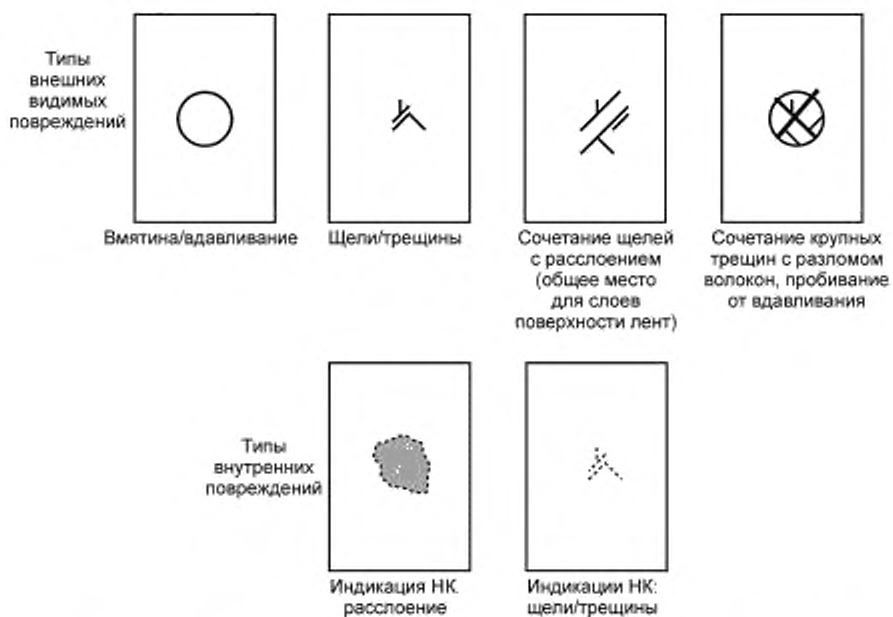
Рисунок 6 — Часто наблюдаемые модели повреждений при поперечном нагружении
