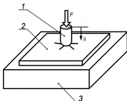
1 — индентор; 2 — образец; 3 — опора; F — контактная нагрузка
