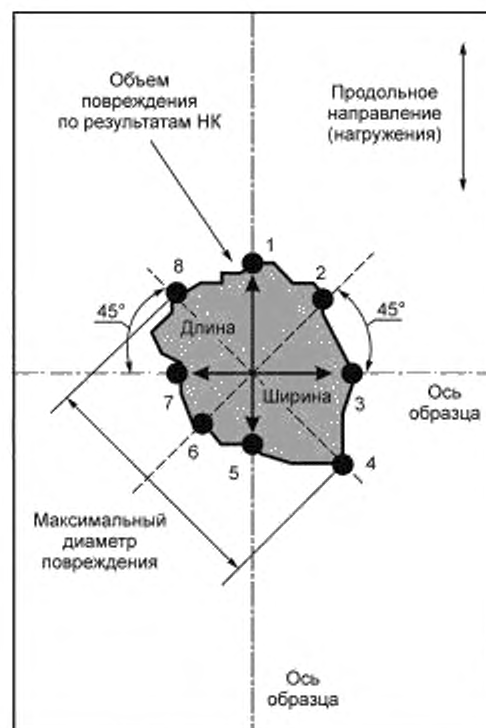
Рисунок 5 — Измерение объема повреждения
