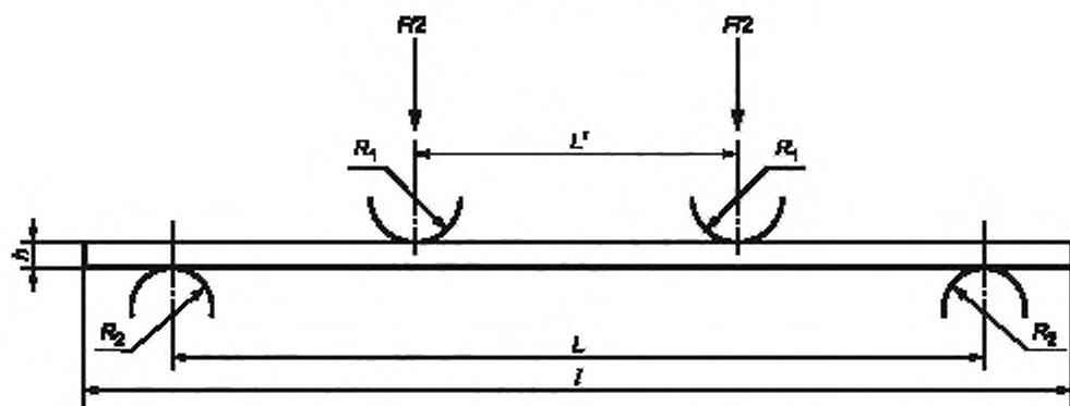
h — толщина образца, R_1 — радиус закругления пуансона, R_2 — радиус закругления краев опор; L — пролет между опорами, L' — пролет между верхними опорами. l — длина образца
