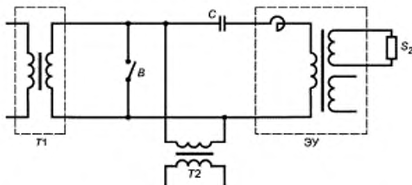
T1 — питающий трансформатор; C — конденсатор отбора мощности емкостного трансформатора; T2 — трансформатор напряжения для осциллографирования; ZU — электромагнитное устройство емкостного трансформатора; B — высоковольтный короткозамыкатель; S_2 — нагрузка основной вторичной обмотки
