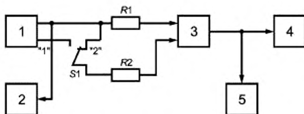
Рисунок 18 — Схема измерения коэффициента асимметрии входа телефонного канала
