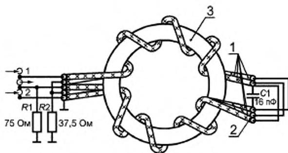
1 — коаксиальный кабель типа РК-75-1,5-22; 2 — коаксиальный кабель типа КВФ-37; 3 — ферритовое кольцо типа 400НН К38×24×7 — 2 шт.; R1 — резистор сопротивлением 75 Ом; R2 — резистор сопротивлением 37,5 Ом; C1 — конденсатор 16 пФ
