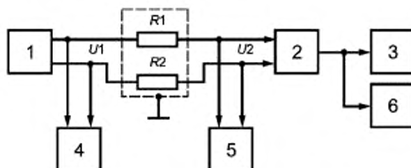
Рисунок 17 — Схема измерения сопротивления симметричного НЧ-входа
