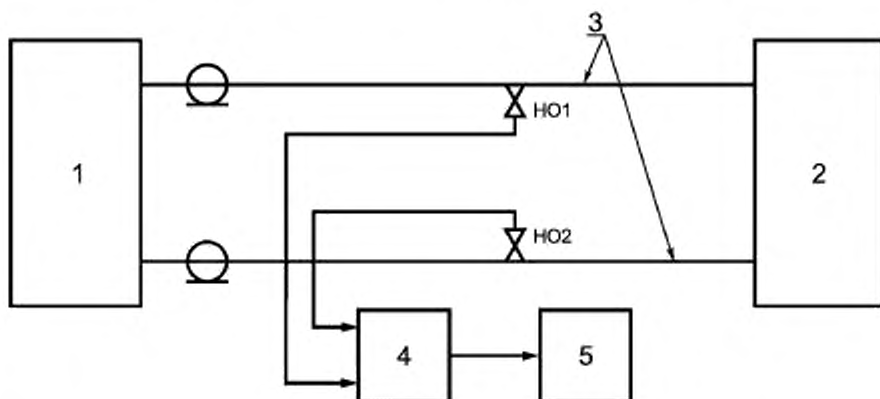
1 — передатчик; 2 — симметричная антенна или ее эквивалент; 3 — двухпроводный коаксиальный симметричный фидер; 4 — сумматор противофазных сигналов; 5 — СИ; HO1, HO2 — направленные ответвители падающих волн
