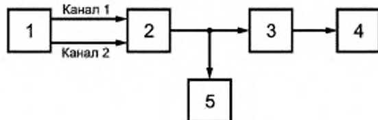
Рисунок 20 — Схема измерения краевых искажений телеграфных сигналов
