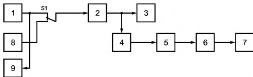
1 — генератор сигналов НЧ; 2 — передатчик; 3 — эквивалент антенны; 4 — элемент связи; 5 — анализатор модуляции (измерительный декодер); 6 — полосовой фильтр; 7 — милливольтметр НЧ; 8 — экранированный резистор сопротивлением (600 \pm 30) Ом; 9 — милливольтметр НЧ
