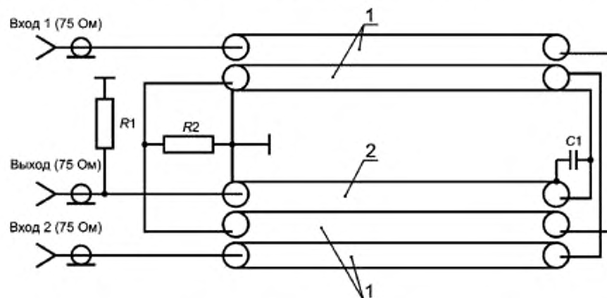
1 — коаксиальный кабель типа РК-75-1,5-22; 2 — коаксиальный кабель типа КВФ-37; R1 — резистор сопротивлением 75 Ом; R2 — резистор сопротивлением 37,5 Ом; C1 — конденсатор 18 пФ
