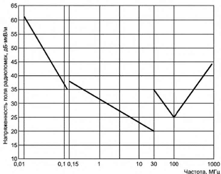
Рисунок 3 — Нормы напряженности поля радиопомех
