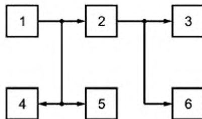
Рисунок 12 — Схема измерения неравномерности АЧХ телефонных каналов
