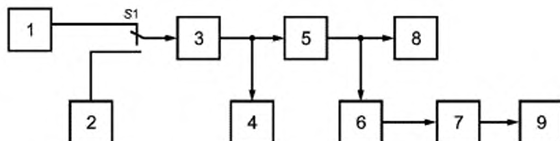
1 — генератор шума; 2 — генератор сигналов НЧ; 3 — формирующий фильтр; 4 — милливольтметр НЧ; 5 — передатчик; 6 — элемент связи; 7 — анализатор спектра ВЧ; 8 — эквивалент антенны; 9 — частотомер; S1 — переключатель
