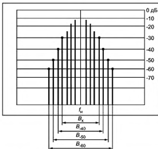
Рисунок 24 — Отсчет контрольной ширины полосы радиочастот ( B_x ) и внеполосных радиокосебаний на анализаторе спектра с логарифмическим детектором
