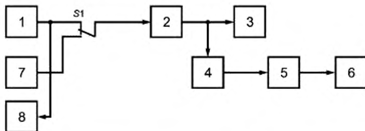
1 — генератор сигналов НЧ; 2 — передатчик; 3 — эквивалент антенны; 4 — элемент связи; 5 — УОП передатчика; 6 — милливольтметр НЧ; 7 — экранированный резистор сопротивлением (600 \pm 30) Ом; 8 — милливольтметр НЧ; S1 — переключатель
