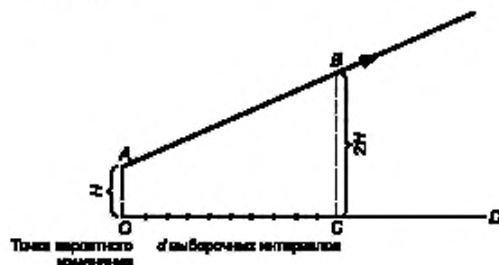
Рисунок Г.1 — Построение локальной разрешающей линии
