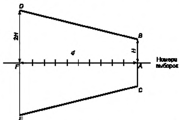
Рисунок 1 — Шаблон усеченной V-маски
