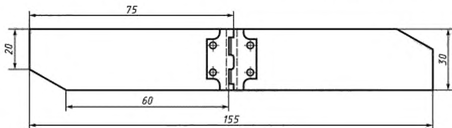
Рисунок Г.1 — Давильная пластина
