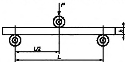
Рисунок 2 — Схема испытания образца
