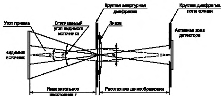
Рисунок 8а — Измерительная установка с изображением источника
