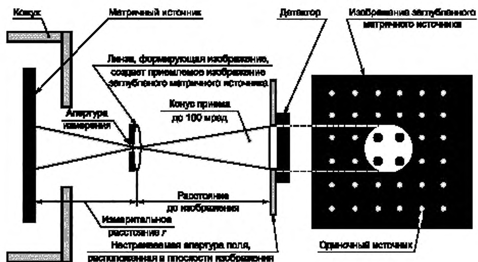
10b -- Геометрия измерения для затлубленного источника
