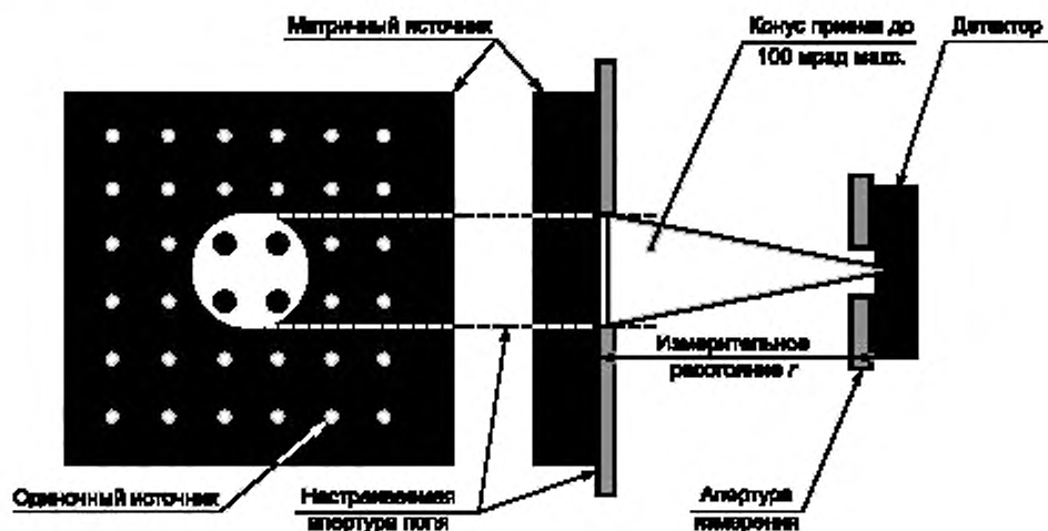
10a -- Геометрия измерения для доступного источника
