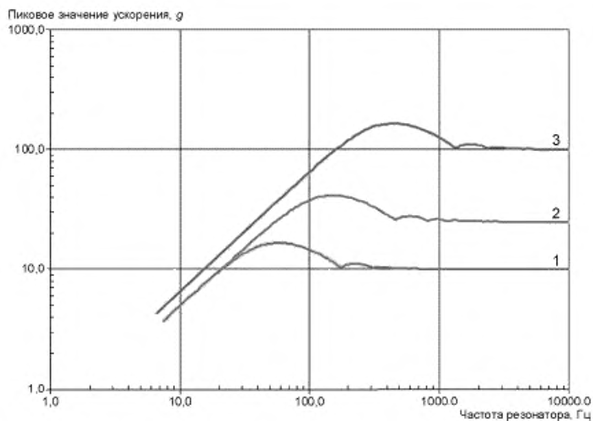
Рисунок 44 — Рекомендованные тестовые воздействия (ударные спектры) для повторяющихся ударов по [17] (число ударов 100 \times 6 = 600 )
