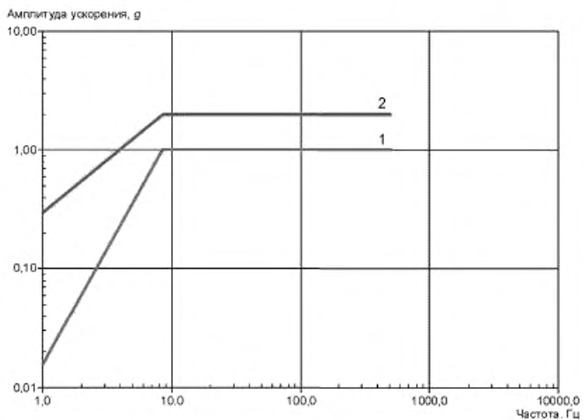
Рисунок 41 — Рекомендуемые тестовые воздействия для гармонической вибрации по [17]
