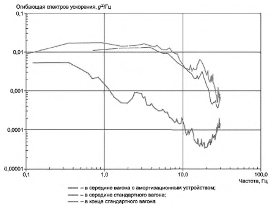
Рисунок 19 — Огибающие спектров для вибрации товарных вагонов в продольном направлении (Американские железные дороги)
