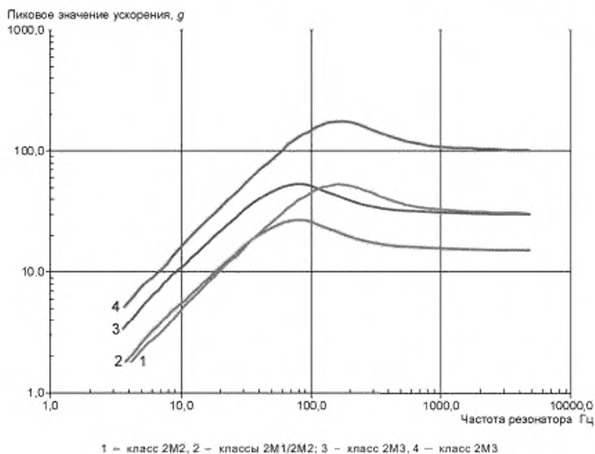
Рисунок 43 — Тестовые воздействия [17] (ударные спектры)
