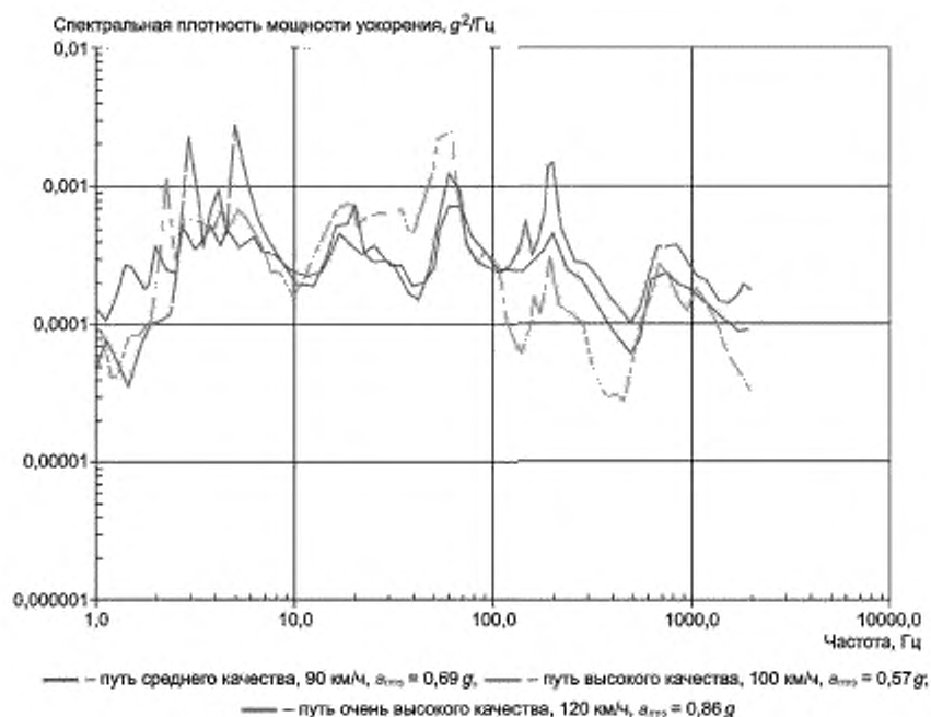
Рисунок 34 — Спектры вибрации в вертикальном направлении для вагонов Французской железной дороги (SNCF) типов А, В и С, по данным [12]
