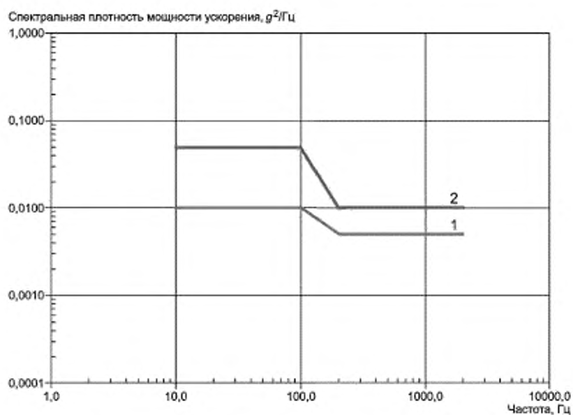
Рисунок 39 — Рекомендованные тестовые воздействия для случайной вибрации по [17] (30 мин по каждой оси, всего — 180 мин)
