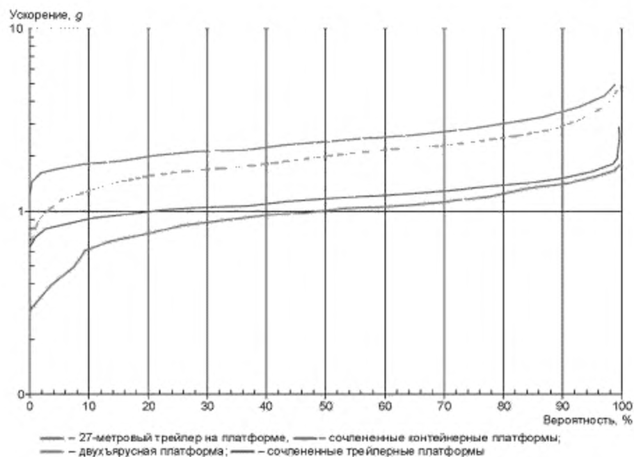
Рисунок 13 — Распределение ускорения в вертикальном направлении при смешанных перевозках (Американские железные дороги)
