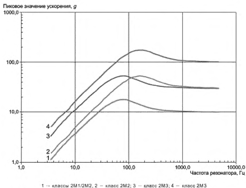
Рисунок 42 — Тестовые воздействия МЭК 60721-3-2:1997 (ударные спектры)
