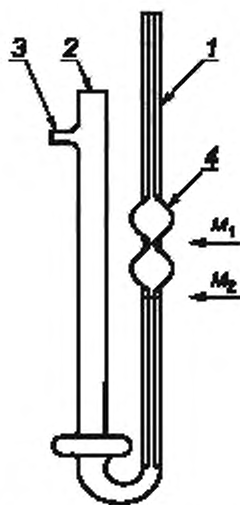
Рисунок В.2.1 — Вискозиметр типа Пинкевича (ВПЖТ-4, ВПЖ-4)
