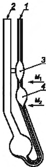
Рисунок В.1 — Вискозиметр типа Канон-Фенске
