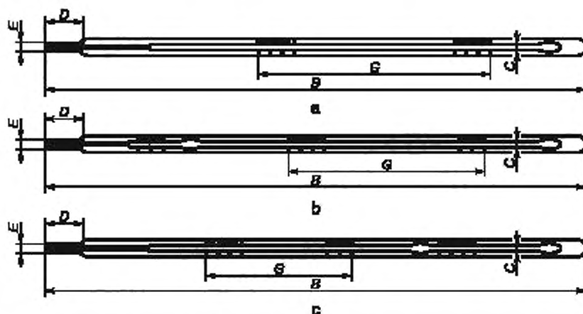
Рисунок Б.1 Различные конструкции термометров
