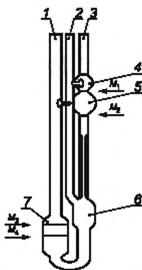
Рисунок В.4 — Вискозиметр типа Убеллоде
