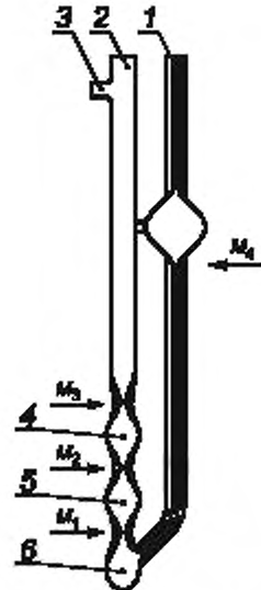
Рисунок В.5 — Вискозиметр типов ВНЖ, ВНЖТ (Канон-Фенске-Опакв)
