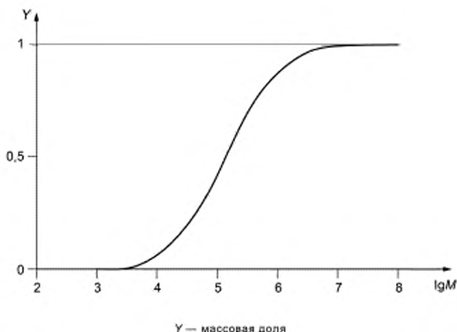
Рисунок 7 — Интегральная кривая молекулярно-массового распределения
