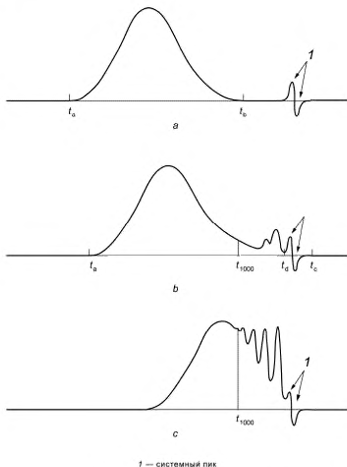
Рисунок 4 — Типичные хроматограммы, получаемые методом ЭХ
