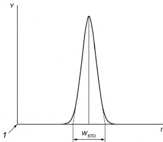
Рисунок 3 — Эксклюзионная хроматограмма стандартного образца с узким молекулярно-массовым распределением
