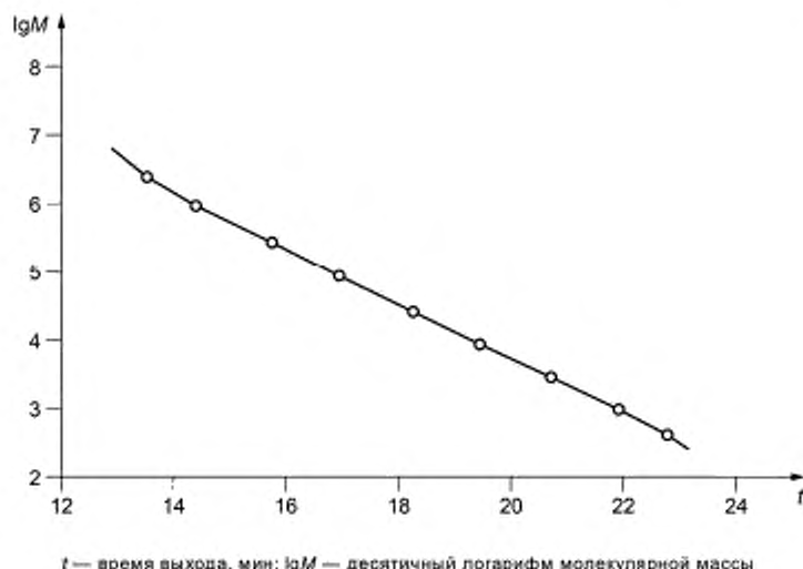
Рисунок 5 — Калибровочная кривая
